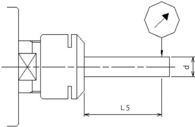
コレットの精度 DIN 6499-A, DIN 6499-B
