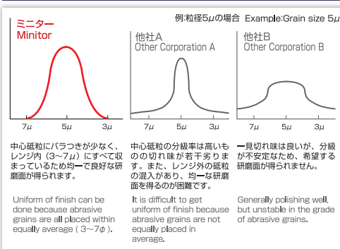
ダイヤモンド砥粒分級曲線 Accuracy of classification curve
