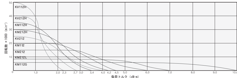
図-4. 回転数 / トルク曲線
